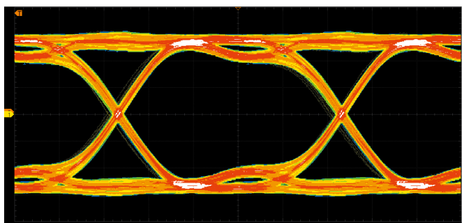
使用750 MHz带宽和1.5 GHz带宽分别对1 Gb/s信号进行眼图观测
